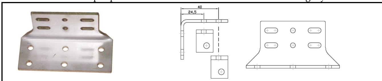
Konzole PAN K 68 - pro protikus F 30
