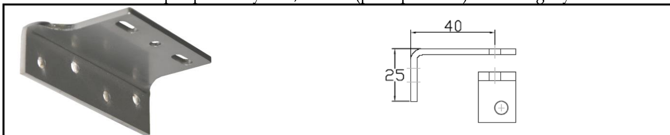
Konzole PAN K 48 - pro protikusy F 10,6 a F 30 (př. Sapa Alure) katalogový kód: 4770048
