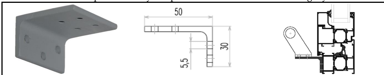
Konzole PAN K 60 - pro čelní uchycení pohonu
