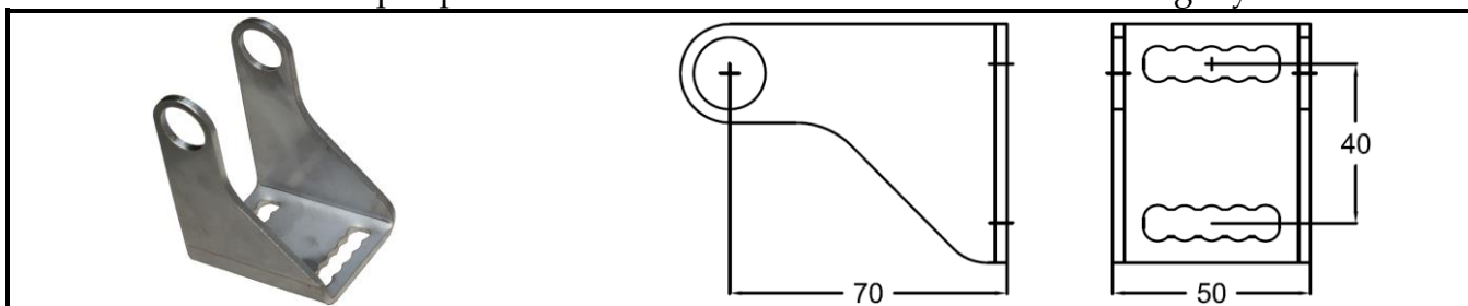
Konzole PAN K 118 - pro pohon LC na světlíku Essmann
