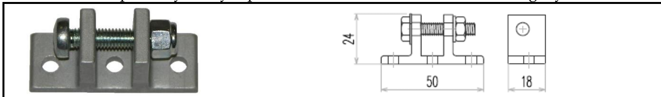
Protikus F 30 - pro uchycení tyče pohonu
