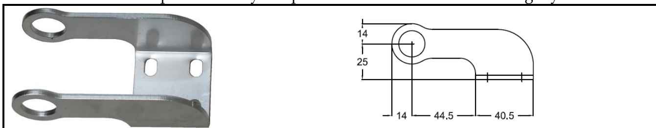
Konzole PAN K 61 - pro čelní uchycení pohonu
