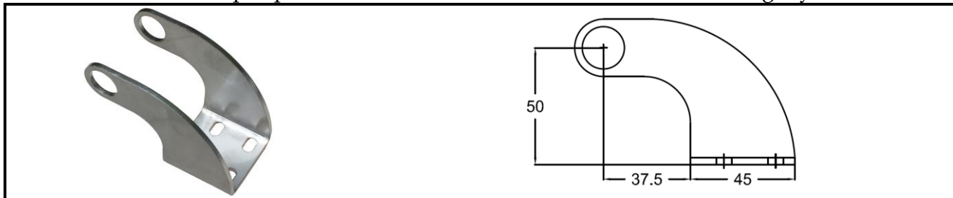
Konzole PAN K 89 - pro pohon LC - nerez
