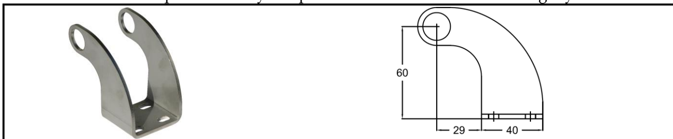
Konzole PAN K 71 - pro čelní uchycení pohonu
