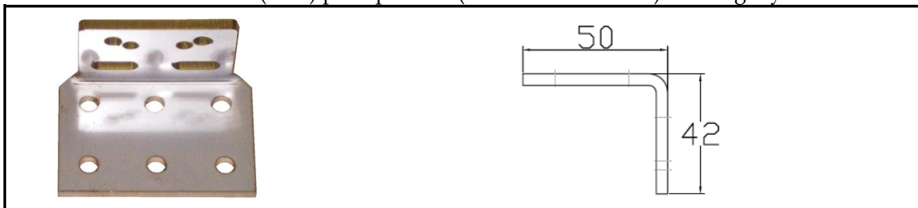
Konzole PAN K 65 - LC (K 30) proti pantům (Schüco AWS 57 RO) katalogový kód: 4770065
