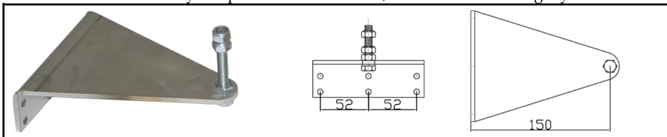
Konzole PAN K 15 - uchycení pohonu na boku okna, šroub M6
