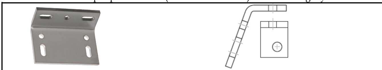
Konzole PAN K 63 - pro protikus F 30 (Schüco AWS 57 RO) katalogový kód: 4770063
