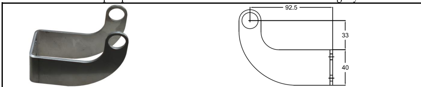
Konzole PAN K 91 - pro pohon LC - nerez
