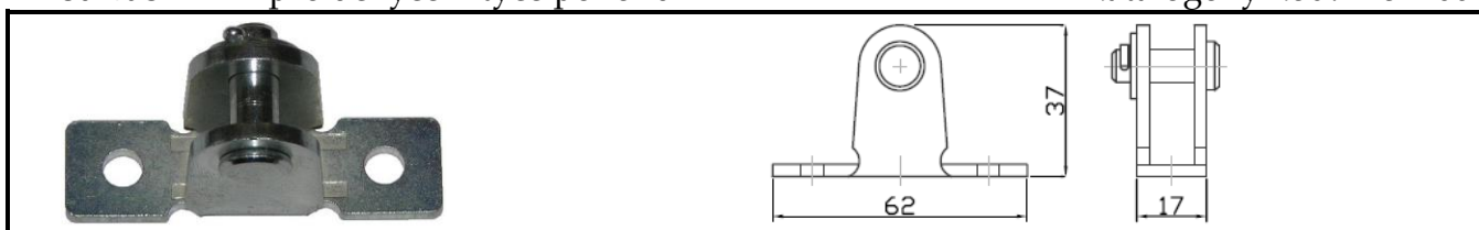
Protikus F 11 - pro uchycení tyče pohonu
