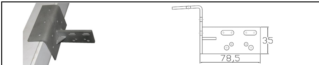
Konzole PAN K 51 - pro pohon LC (konzoli K 30) na boku bodového světlíku
